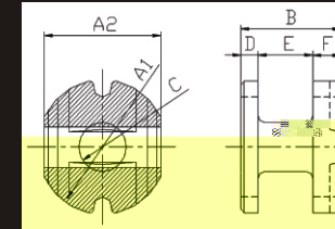
FIG(1) DRC-A1-A2xB-EL
